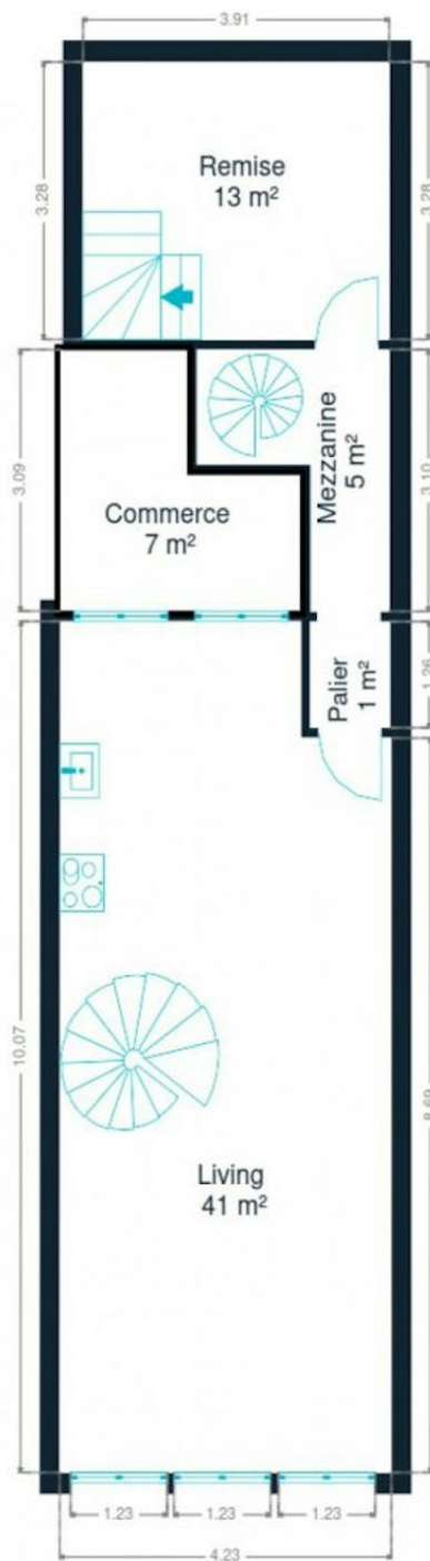
1er étage
